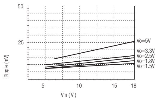
Ripple Vs Vin (Full Load)
